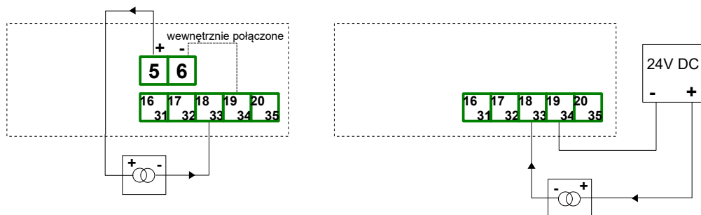
Rys. 4.12. Podłączenia przetworników prądowych 2 przewodowych
