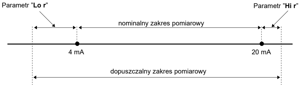
Rys. 6.1. Definicja zakresów pomiarowych w trybie 4 \div 20\text{mA}
