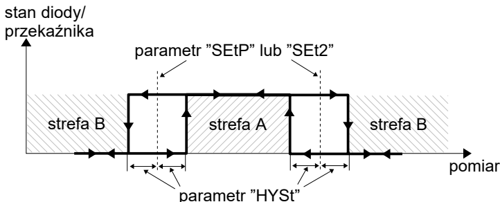
Rys. 6.5. Sterowanie dwuprogowe wyjścia przekaźnikowego / diody LED
