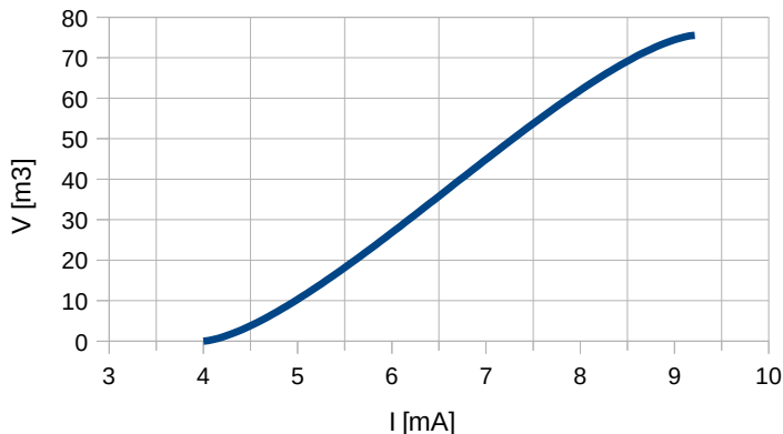
Rys. 10.7 Charakterystyka objętości zbiornika w zależności od prądu wejściowego z sondy poziomego cieczy w zbiorniku (dla zakresu 4÷20mA).
