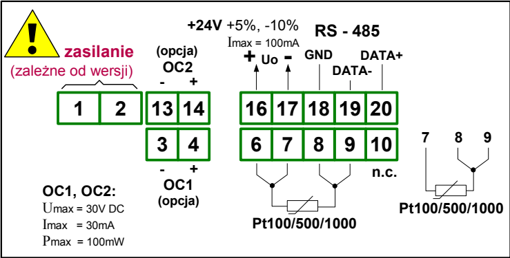
Rys. 4.6. Opis wyprowadzeń dla wersji z wyjściami OC
