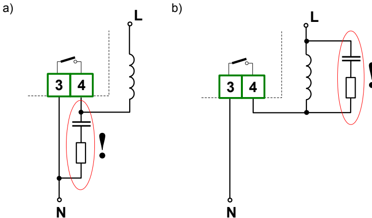
Rys. 4.8. Przykłady równoległego podłączenia obwodu tłumiącego: a) do styków przełącznika; b) do obciążenia indukcyjnego
