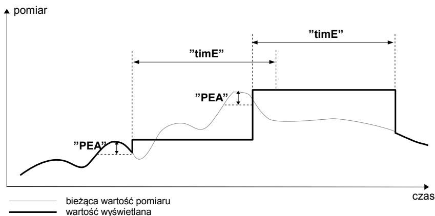
Rys. 6.1. Sposób detekcji wartości szczytowych
