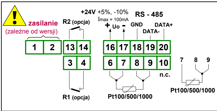
Rys. 4.5. Opis wyprowadzeń dla wersji z wyjściami przekąźnikowymi
