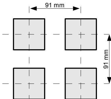
Rys. 4.3. Montaż wielu urządzeń
