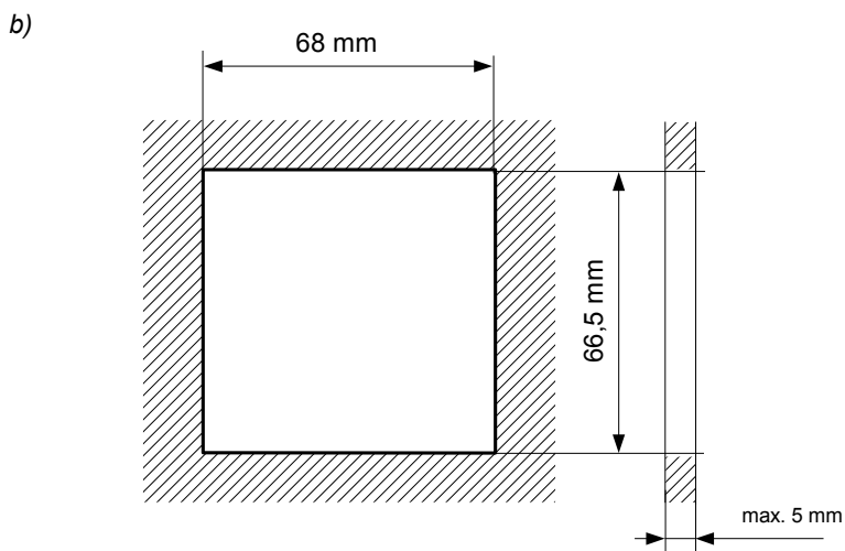
Rys. 4.1. Wymiary montażowe: a) zalecane, b) dopuszczalne
