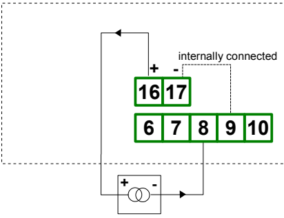
Rys. 4.7. Podłączenia przetworników prądowych 2 przewodowych
