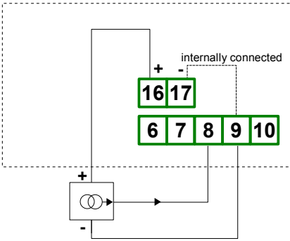
Rys. 4.8. Podłączenia przetworników prądowych 3 przewodowych
