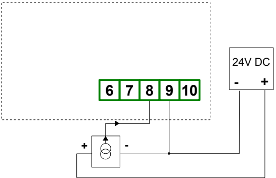
Rys. 4.8. Podłączenia przetworników prądowych 3 przewodowych
