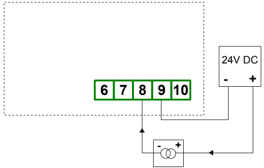
Rys. 4.7. Podłączenia przetworników prądowych 2 przewodowych
