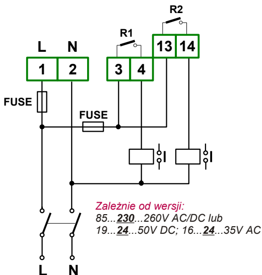
Rys. 4.10. Podłączenie zasilania oraz przełączników sterujących obciążeniami
