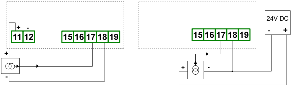
Rys. 4.14. Podłączenia przetworników prądowych 3 przewodowych
