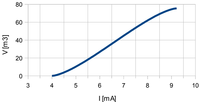
Rys. 9.7 Charakterystyka objętości zbiornika w zależności od prądu wejściowego z sondy poziomego cieczy w zbiorniku (dla zakresu 4÷20mA).
