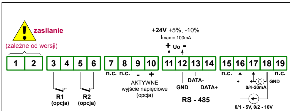
Rys. 4.11. Opis wyprowadzeń dla wersji z wyjściami przekąźnikowymi oraz aktywnym wyjściem napięciowym
