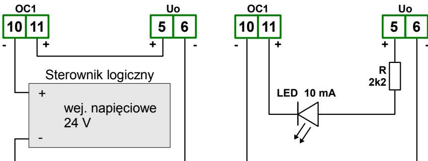
Rys. 4.18. Przykładowe podłączenia wyjścia typu OC (tylko dla urządzeń posiadających wyjście typu OC)
