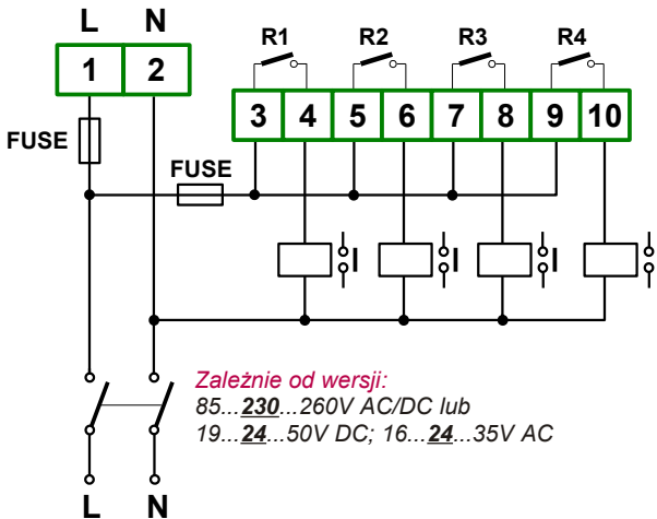
Rys. 4.16. Podłączenie zasilania oraz przekaźników sterujących obciążeniami
