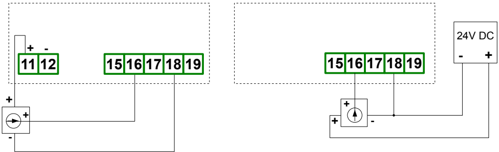
Rys. 4.15. Podłączenia przetworników napięciowych
