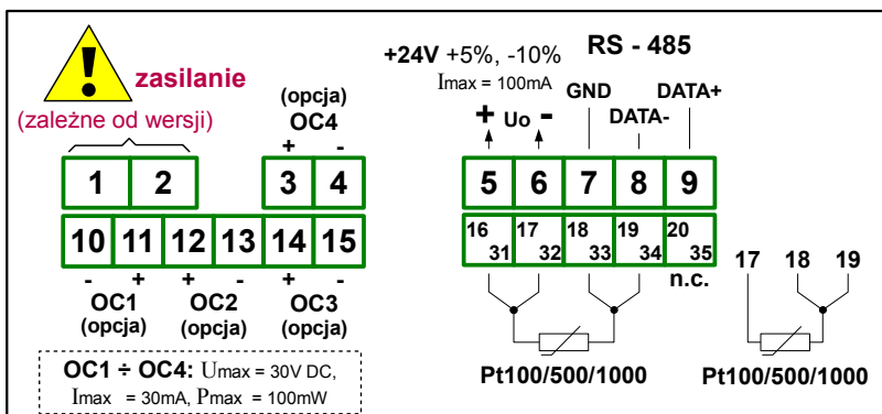
Rys. 4.7. Opis wyprowadzeń dla wersji z wyjściami typu OC
