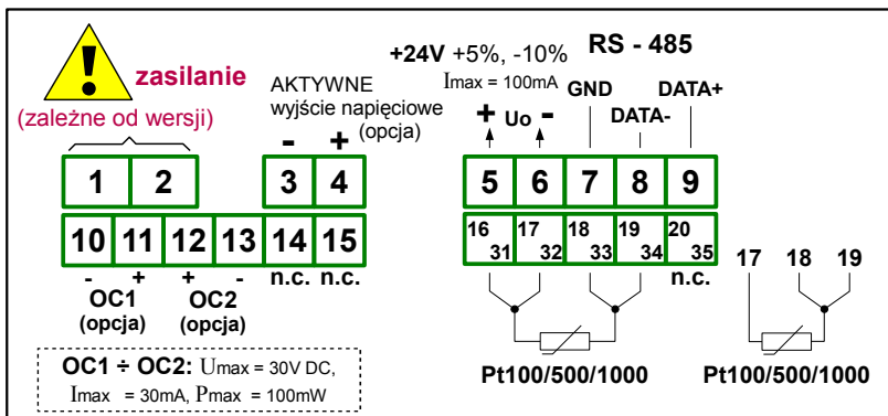
Rys. 4.13. Opis wyprowadzeń dla wersji z wyjściami typu OC oraz aktywnym wyjściem napięciowym
