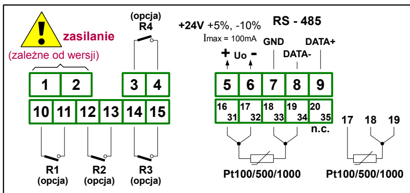
Rys. 4.6. Opis wyprowadzeń dla wersji z wyjściami przekaźnikowymi
