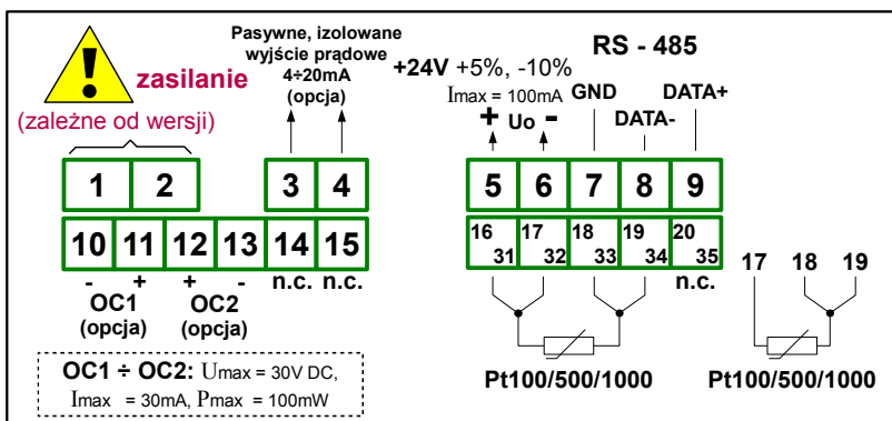
Rys. 4.11. Opis wyprowadzeń dla wersji z wyjściami typu OC oraz pasywnym wyjściem prądowym
