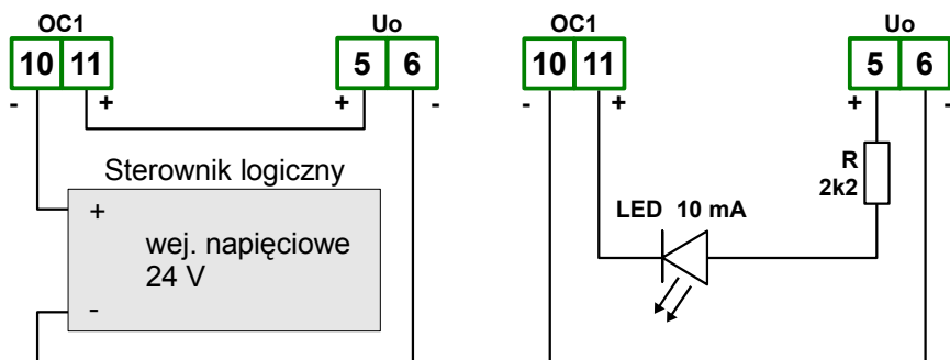
Rys. 4.17. Przykładowe podłączenia wyjścia typu OC (tylko dla urządzeń posiadających wyjście typu OC)
