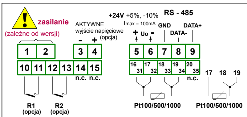
Rys. 4.12. Opis wyprowadzeń dla wersji z wyjściami przekaźnikowymi oraz aktywnym wyjściem napięciowym
