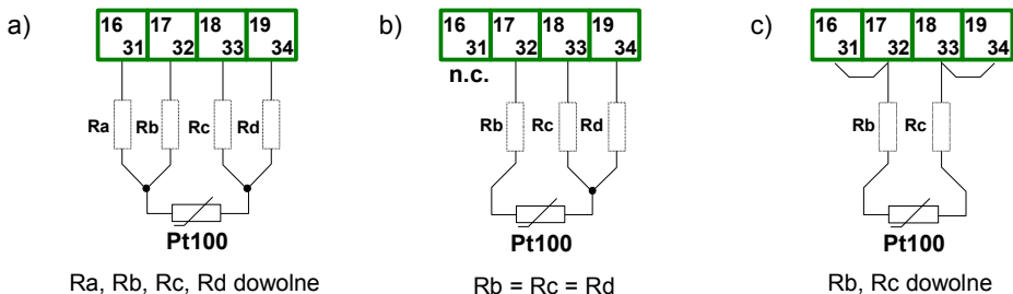
Rys. 4.14. Podłączenia zewnętrzne czujników: a) 4-przewodowe; b) 3-przewodowe; c) 2-przewodowe
