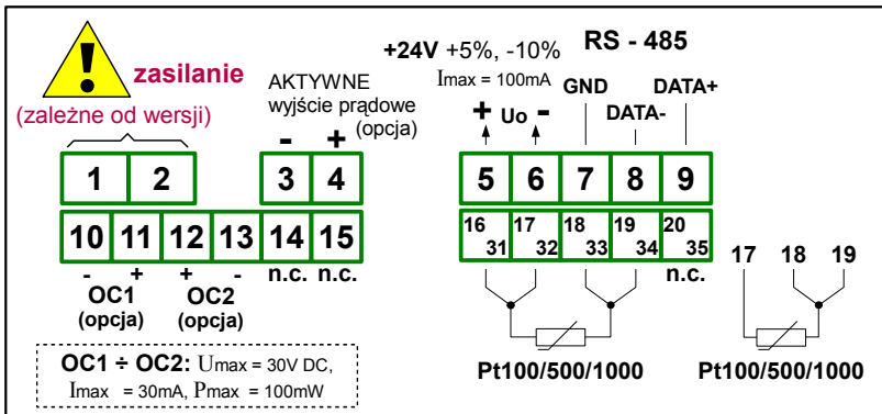
Rys. 4.9. Opis wyprowadzeń dla wersji z wyjściami typu OC oraz aktywnym wyjściem prądowym
