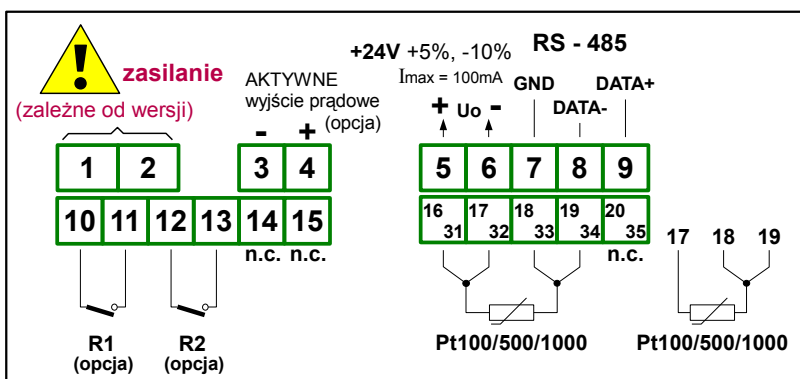
Rys. 4.8. Opis wyprowadzeń dla wersji z wyjściami przekaźnikowymi oraz aktywnym wyjściem prądowym
