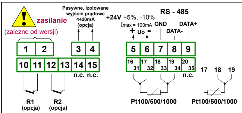
Rys. 4.10. Opis wyprowadzeń dla wersji z wyjściami przekaźnikowymi oraz pasywnym wyjściem prądowym
