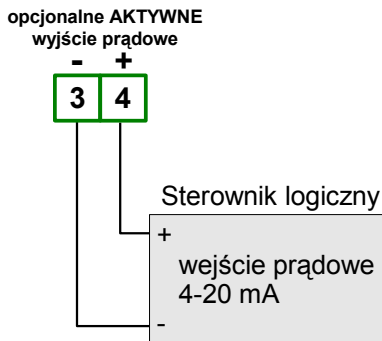
Rys. 4.12. Przykład podłączenia wyjścia prądowego (tylko dla urządzeń posiadających wyjście prądowe)
