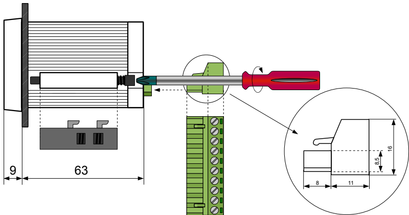
Rys. 4.3. Mocowanie za pomocą uchwytów
