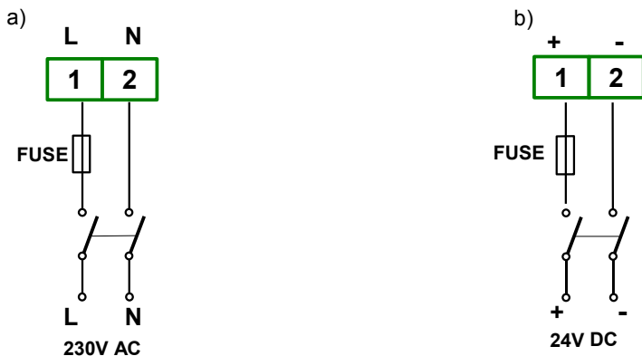
Rys. 4.7. Podłączenie zasilania a) dla wersji 230V AC; b) dla wersji 24V DC
