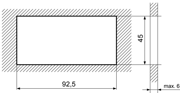
Rys. 4.2. Dopuszczalne wymiary montażowe
