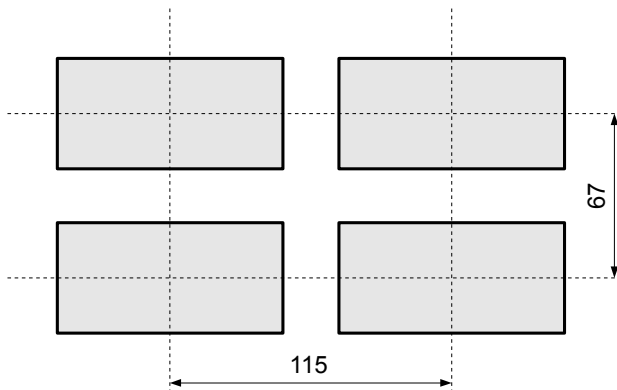
Rys. 4.3. Mocowanie za pomocą uchwytów
