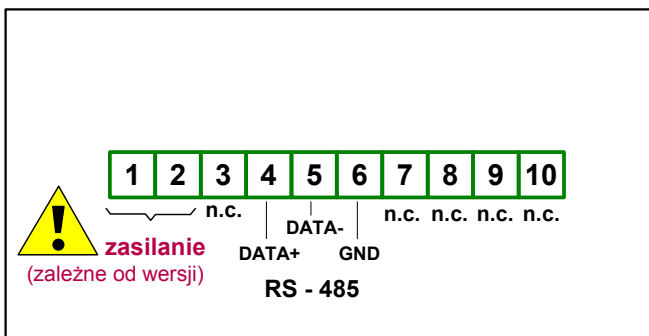
Rys. 4.6. Sposób podłączeń
