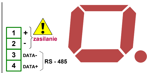
Rys. 4.3. Opis wyprowadzeń
