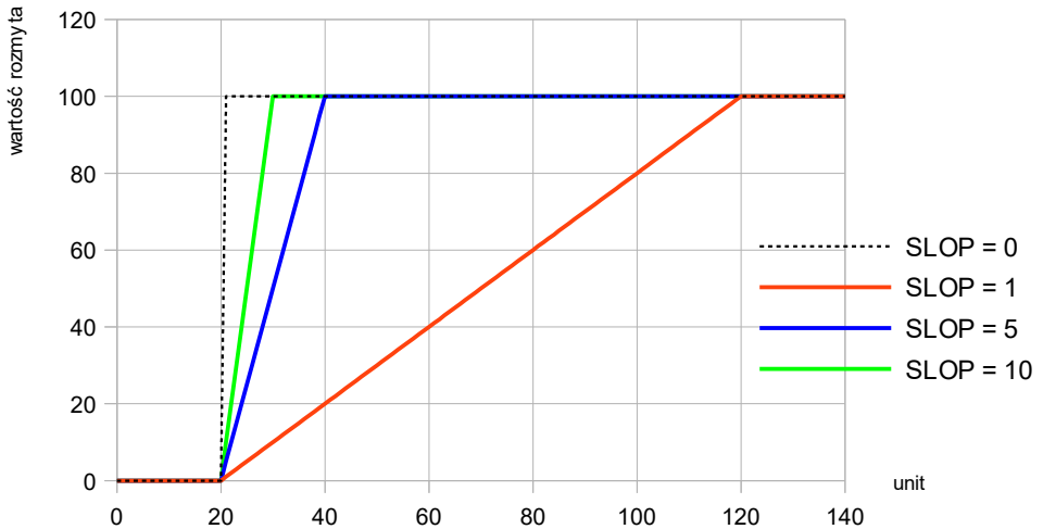
Rys. 7.4. Zmiana rozmytej wartości zadanej w zależności od ustawienia parametru SLOP
