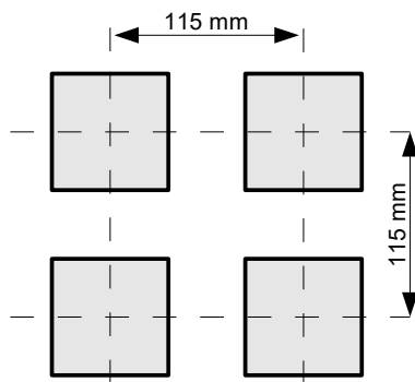
Rys. 4.4. Montaż wielu urządzeń
