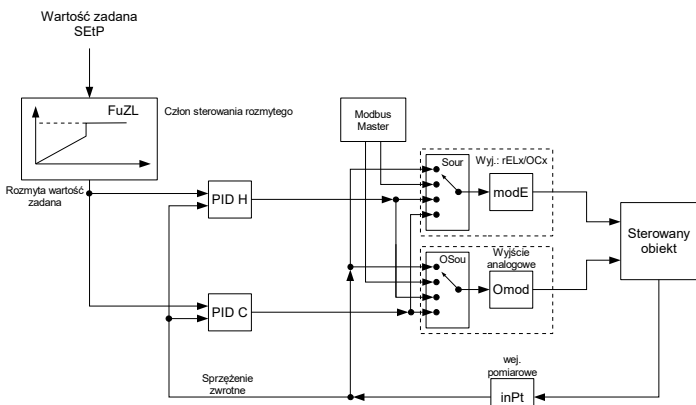
Rys. 6.5 Struktura ogólna urządzenia PUR-99
