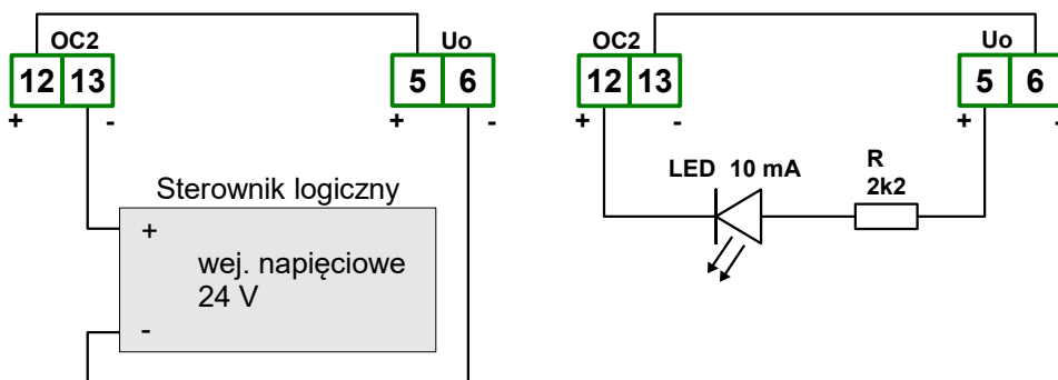
Rys. 4.19. Przykładowe podłączenia wyjścia typu OC (tylko dla urządzeń posiadających wyjście typu OC)
