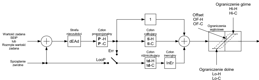
Rys. 6.6. Ogólny schemat regulatora PID zaimplementowanego w urządzeniu PUR-99
