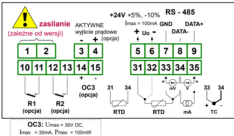
Rys. 4.10. Opis wyprowadzeń dla wersji z dwoma wyjściami przekaźnikowymi, jednym wyjściem typu OC oraz aktywnym wyjściem prądowym
