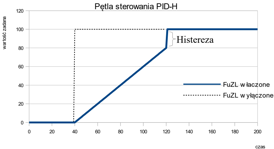
Rys. 6.8. Porównanie odpowiedzi regulatora PID-H na zmianę wartości zadanej przy wykorzystaniu i bez wykorzystania logiki rozmytej
