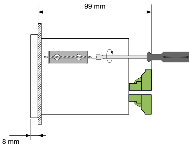
Rys. 4.3. Mocowanie za pomocą uchwytów
