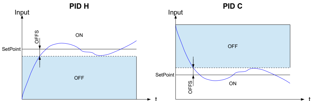
Rys. 6.7. Charakterystyki sterowania przekaźnika w zależności od trybu pracy
