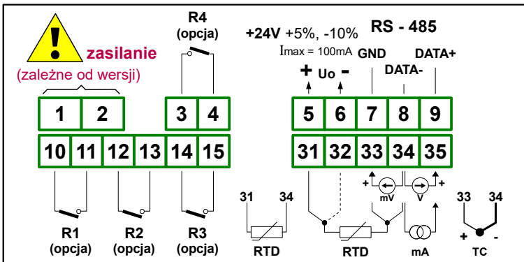
Rys. 4.8. Opis wyprowadzeń dla wersji z czterema wyjściami przekąźnikowymi
