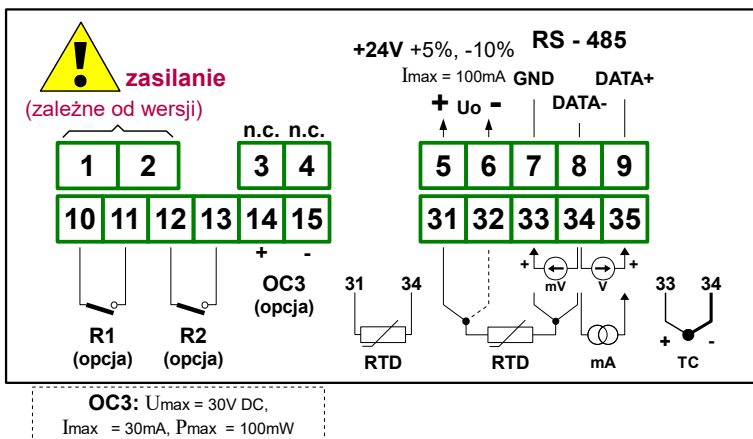
Rys. 4.9. Opis wyprowadzeń dla wersji z dwoma wyjściami przekaźnikowymi oraz wyjściem typu OC
