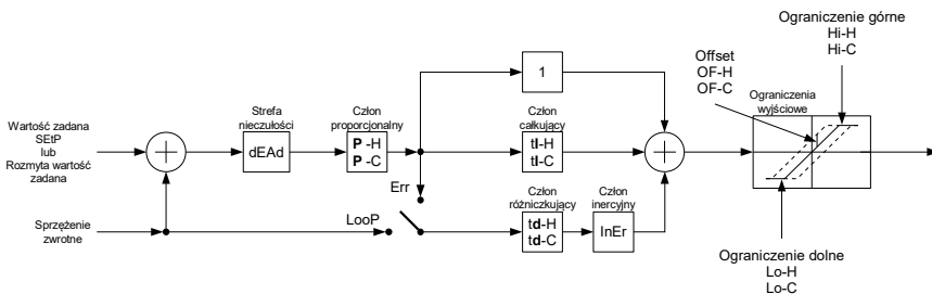
Rys. 7.2. Ogólny schemat regulatora PID zaimplementowanego w urządzeniu PUR-99
