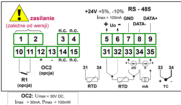
Rys. 4.7. Opis wyprowadzeń dla wersji z wyjściem przekąźnikowym i wyjściem typu OC
