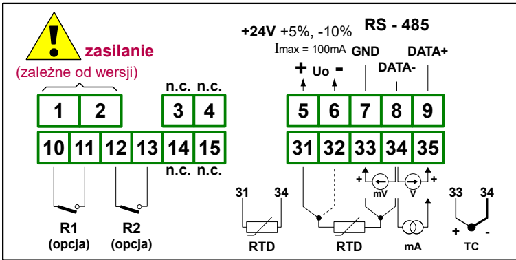
Rys. 4.6. Opis wyprowadzeń dla wersji z dwoma wyjściami przekąźnikowymi
