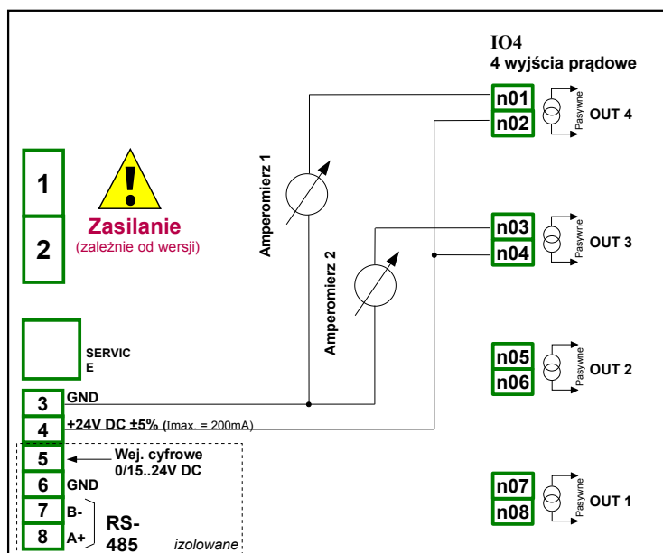
Rys. 8.16. Podłączenia dla Pasywnego wyjścia prądowego od strony zasilania
