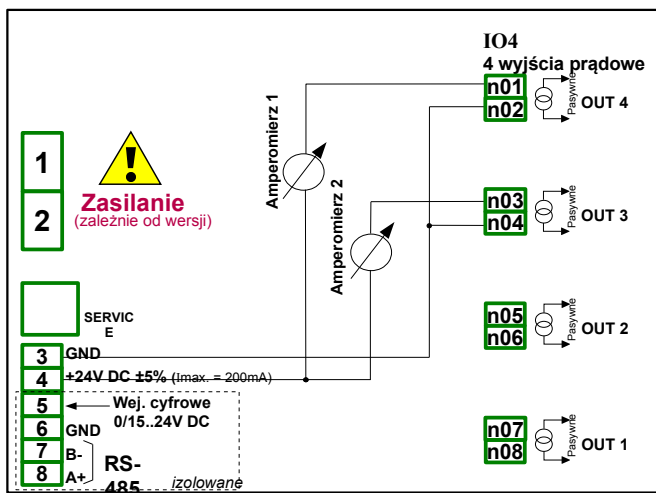
Rys. 7.100. Przykładowy sposób podłączenia pasywnego wyjścia prądowego
