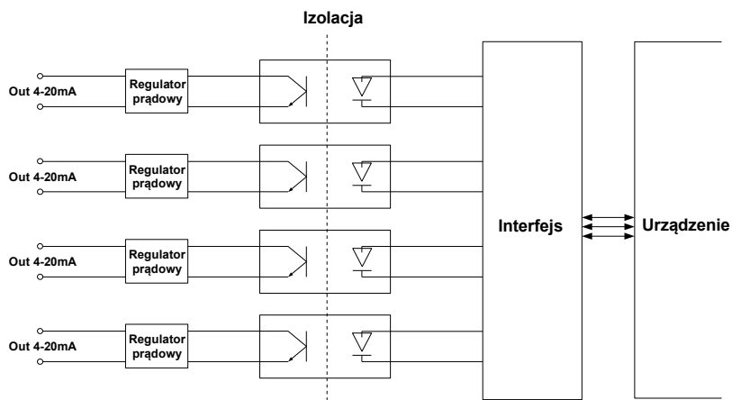
Rys. 8.17. Struktura wewnętrzna modułów wyjść prądowych
