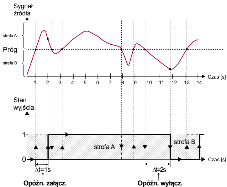
Rys. 7.91. Zasada pracy wyjść przełącznikowych dla przykładowych ustawień czasowych: Opóźn.załącz. = 1 sec., Opóźn.wyłącz. = 2 sec.
