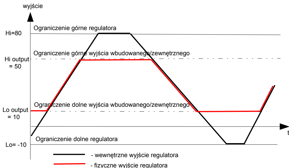
Rys. 7.111. Ograniczenia wyjścia pętli sterującej
