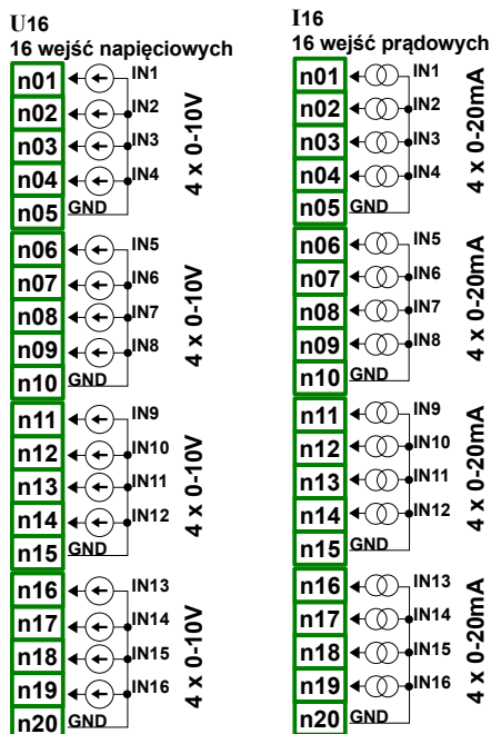
Rys. 4.9. Moduły wejść prądowych i napięciowych
