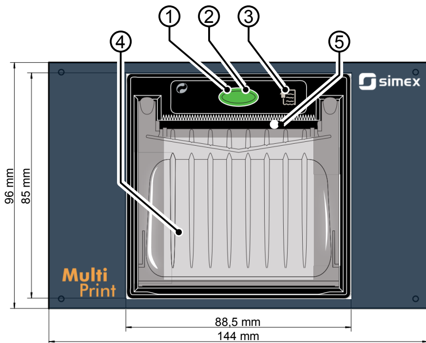
Rys. 8.19. Widok płyty czołowej
