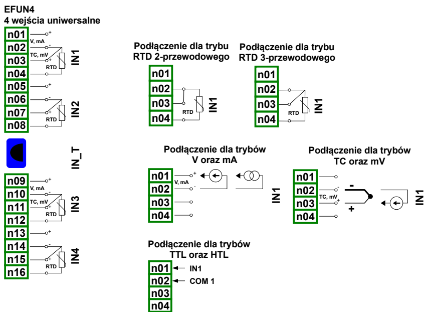
Rys. 8.10. Moduły wejść uniwersalnych
