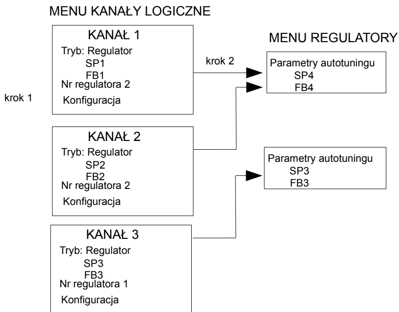
Rys. 7.110. Schemat konfiguracji Regulatora z poziomu menu Kanały logiczne
