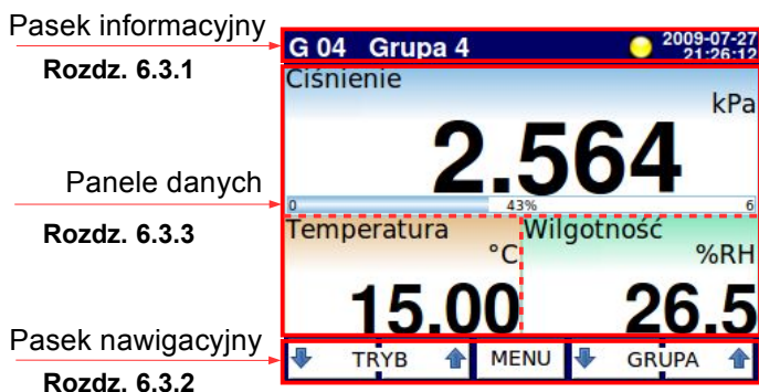
Rys. 6.4. Widok wyświetlacza MultiCon CMC-99 Lite po dotknięciu ekranu w czasie normalnej pracy urządzenia
