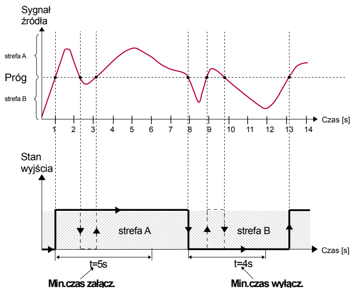
Rys. 7.92. Zasada pracy wyjść przełącznikowych dla przykładowych ustawień czasowych: Min.czas załącz. = 5 sec., Min.czas wyłączy. = 4 sec.
