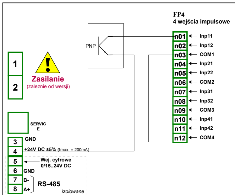
Rys. 7.81. Schemat podłączeniowy modułu FP4 i czujnika typu PNP
