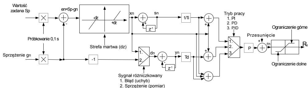
Rys. 7.107. Schemat blokowy Regulatora zaimplementowanego w urządzeniu
