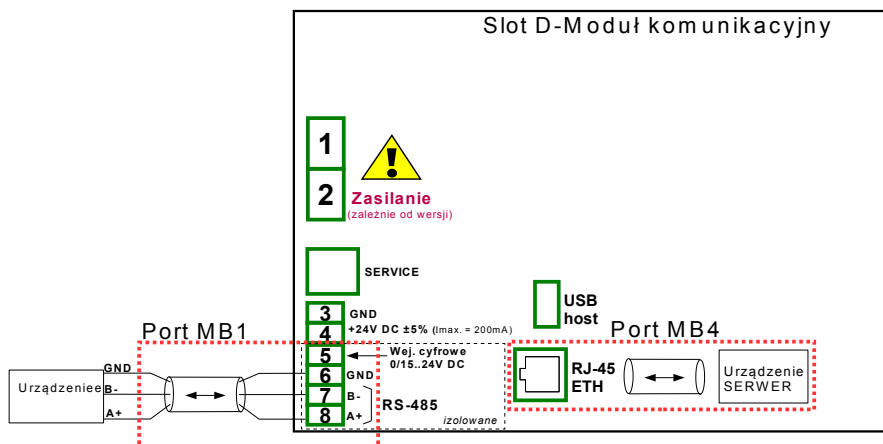
Rys. 7.133. Szeregowe porty komunikacyjne dostępne w urządzeniu
