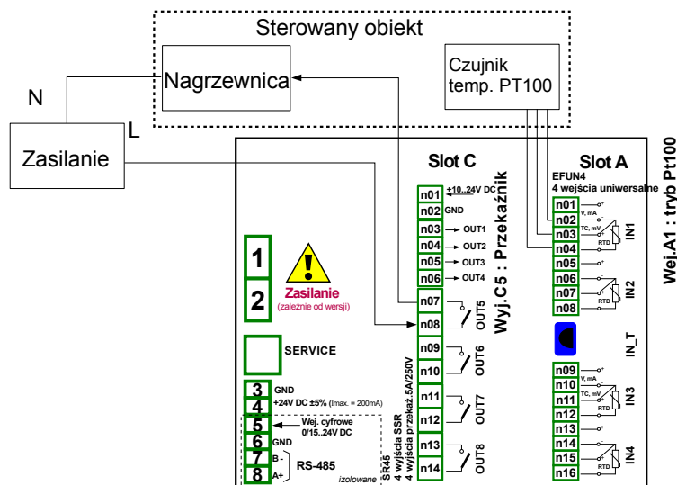
Rys. 7.99. Przykładowy sposób podłączenia do wejścia RTD i wyjścia przełącznikowego
