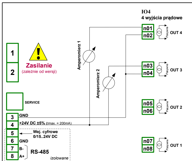
Rys. 8.15. Podłączenia dla Pasywnego wyjścia prądowego od strony GND
