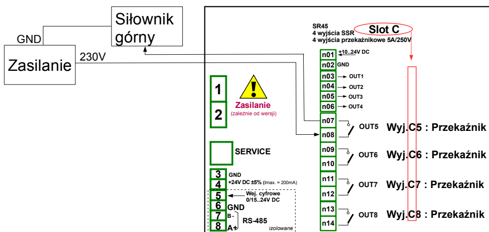
Rys. 7.78. Schemat połączeniowy dla modułu SR45
