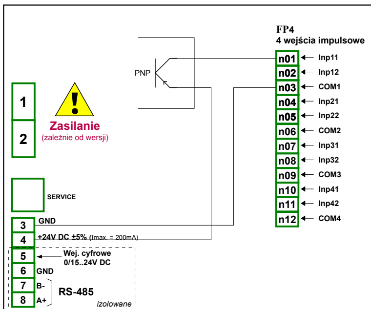
Rys. 8.8. Schemat połączeniowy dla modułu FP4 i czujnika typu PNP
