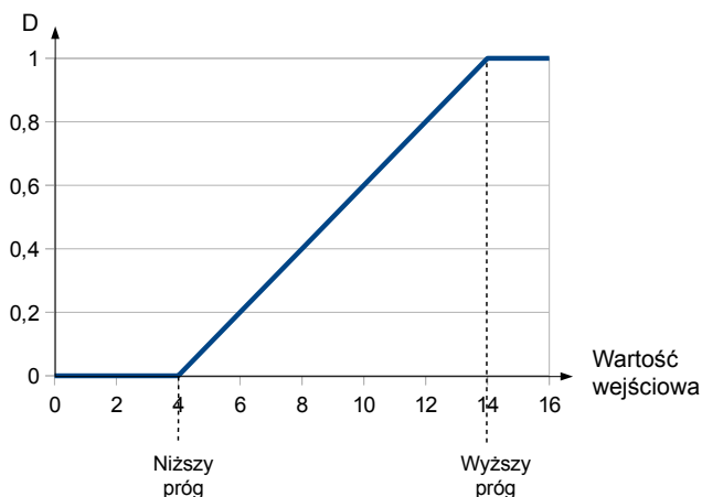
Rys. 7.94. Charakterystyka wejściowo - wyjściowa sygnału w trybie PWM dla parametrów: Niższy próg=4, Wyższy próg=14
