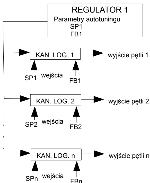
Rys. 7.108. Ogólny schemat konfiguracji Regulatora z wykorzystaniem autotuningu
