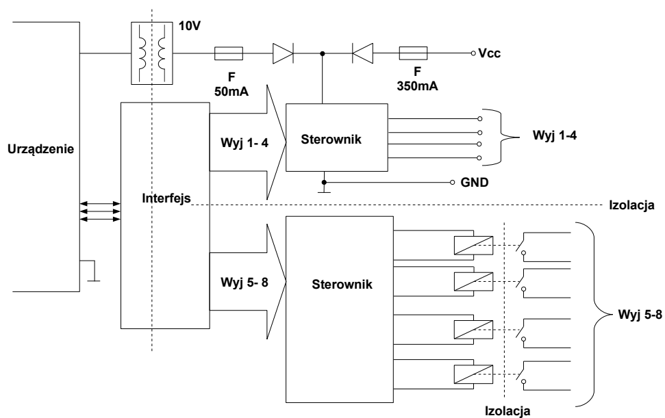
Rys. 8.13. Struktura wewnętrzna mieszanego modułu z przekaźnikami
