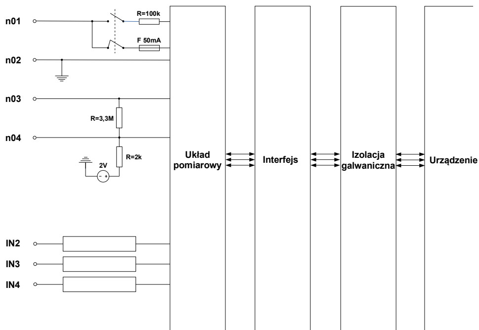
Rys. 8.11. Struktura wewnętrzna modułu wejść uniwersalnych EFUN4
