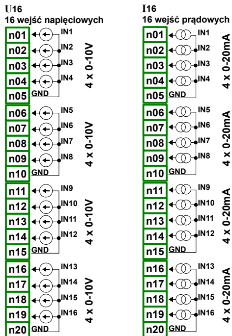
Rys. 8.2. Moduły napięciowe i prądowe
