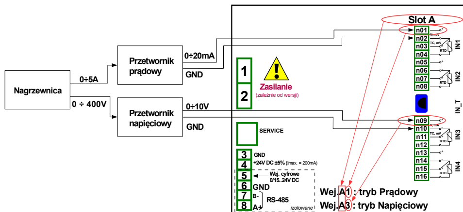
Rys. 7.72. Schemat połączeniowy dla modułu EFUN4
