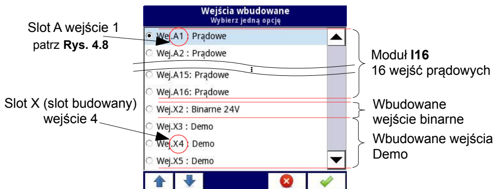
Rys. 7.83. Przykładowa konfiguracja urządzenia z dostępnymi wejściami wbudowanymi
