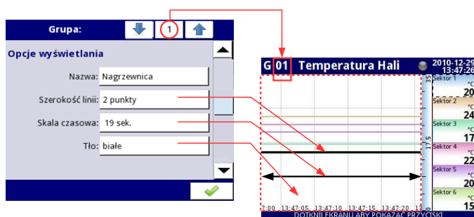
Rys. 7.123. Przykładowe ustawienia parametrów Grupy - wszystkie Sloty ustawione na Kanale logicznym
