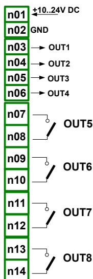
Rys. 8.12. Mieszane moduły wyjść przełącznikowych
