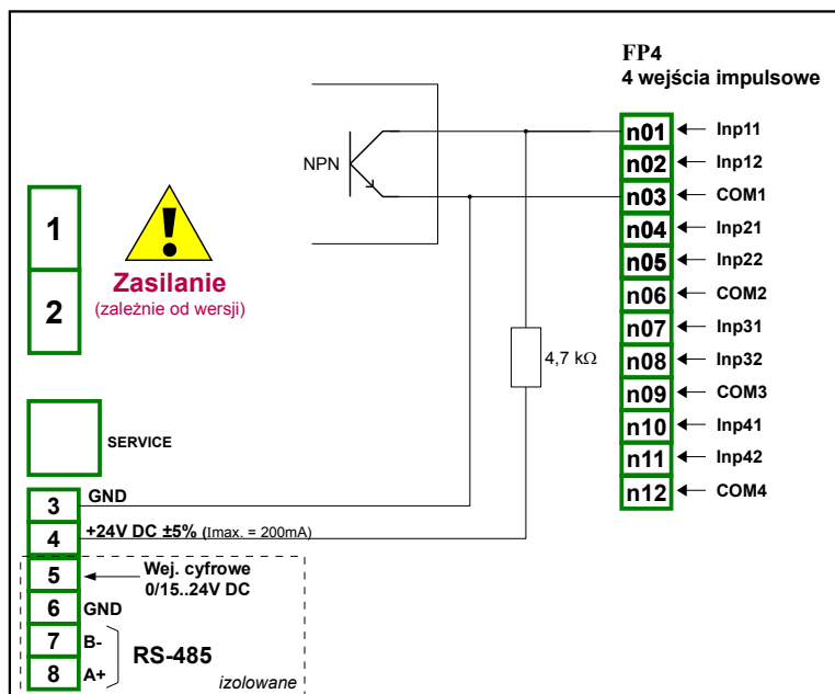
Rys. 8.9. Schemat połączeniowy dla modułu FP4 i czujnika typu NPN
