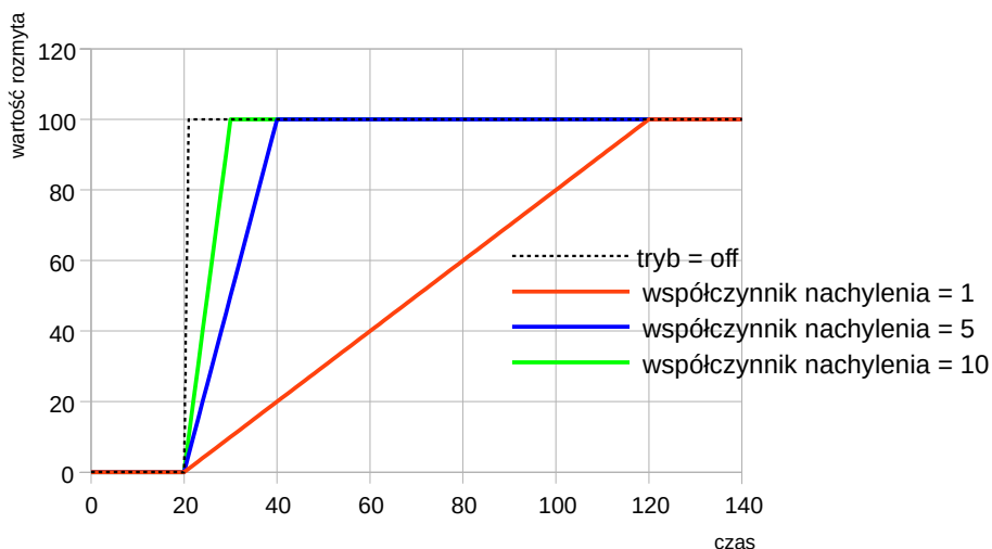
Rys. 7.104. Zmiana rozmytej wartości zadanej w zależności od ustawienia parametru Współczynnik nachylenia
