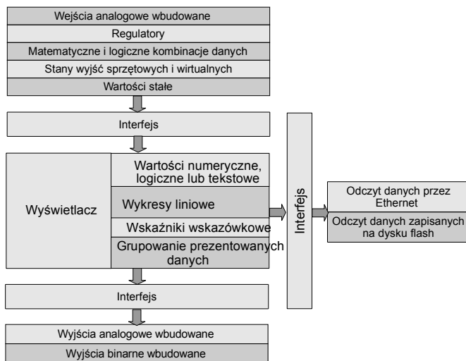
Rys. 2.1. Ogólna charakterystyka urządzenia
