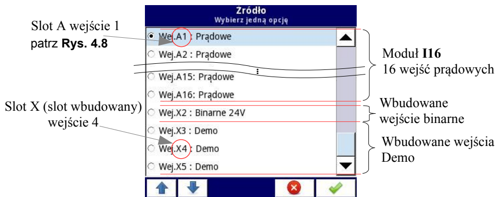
Rys. 7.58. Przykładowe opcje dla Źródła w trybie Wejście sprzętowe
