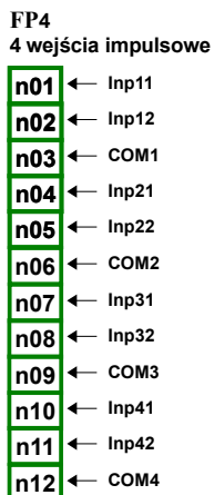
Rys. 8.7. Moduły przepływomierzowe
