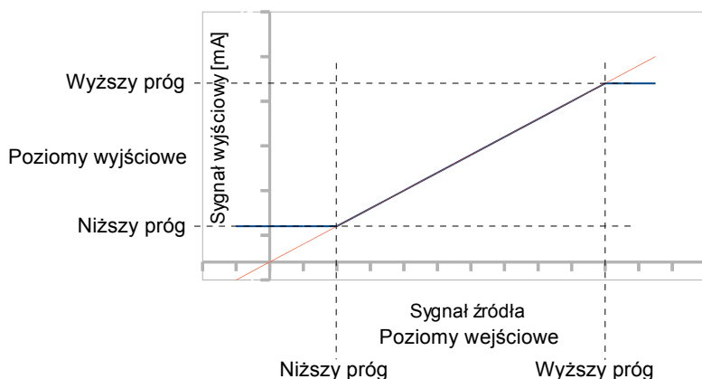
Rys. 7.97. Zależność sygnału wyjściowego (niebieski) od wejściowego (czerwony) dla Wyjścia prądowego
