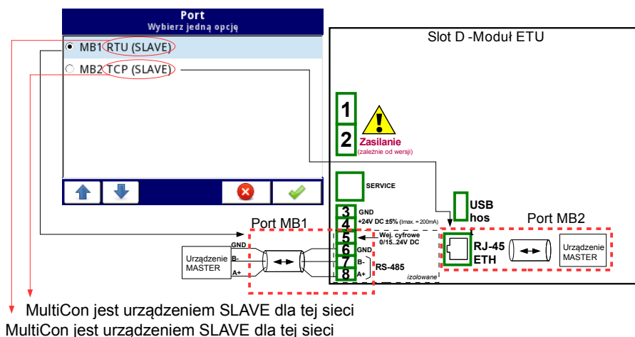
Rys. 7.63. Przykładowe podłączenie urządzenia MultiCon CMC-99 Lite w sieci z podglądem skonfigurowanych portów Modbus
