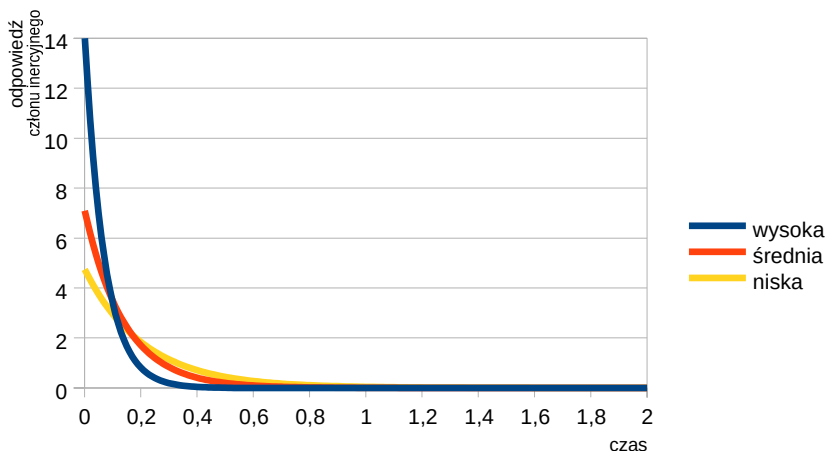
Rys. 7.103. Odpowiedzi układu inercyjnego w zależności od współczynnika T
