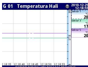
Rys. 7.125. Przykładowe ustawienia parametrów Grupy - Sloty ustawione na Kanale logicznym oraz nieaktywne
