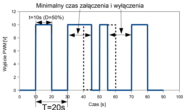
Rys. 7.95. Przykładowy przebieg wyjściowy przełącznika SSR w trybie PWM
