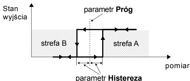
Rys. 7.88. Sterowanie jednoprogowe wyjścia przełącznikowego
