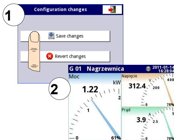
Rys. 7.77. Widok okna po zapisie konfiguracji
