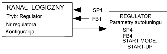
Rys. 7.115. Ustawienia automatycznego startu autotuningu
