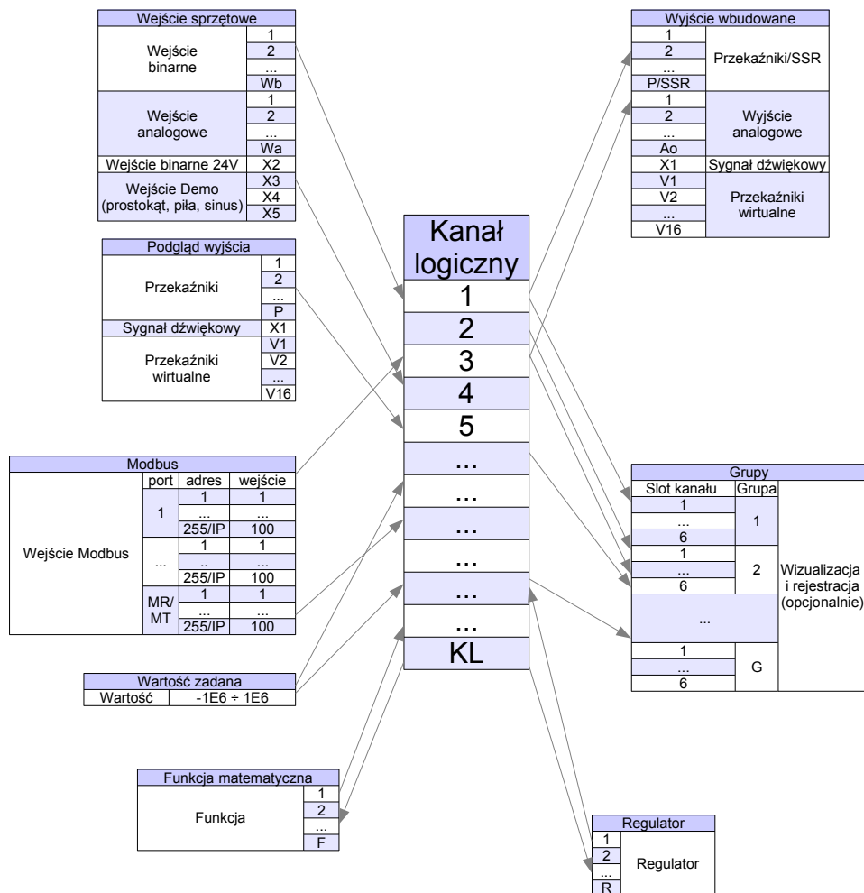
Rys. 5.1. Ogólna struktura powiązań kanału logicznego z wejściami i wyjściami urządzenia
