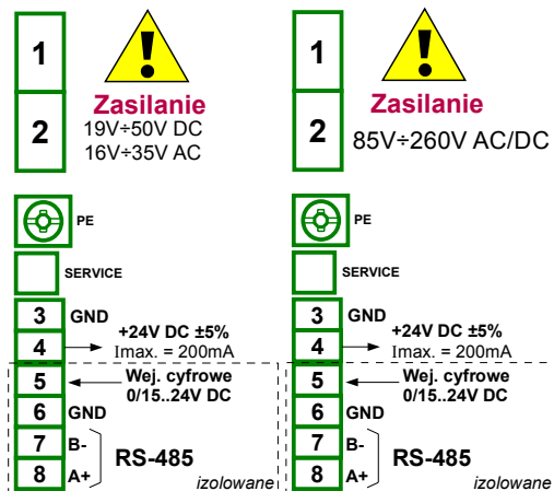
Rys. 8.1. Moduły zasilające (od lewej): PS32, PS42
