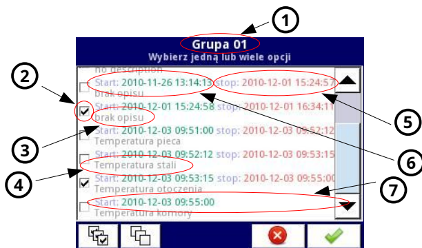
Rys. 7.21. Przykładowy widok okna wyboru plików rejestracji danych dla grupy 1
