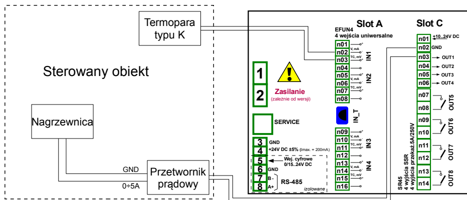
Rys. 7.116. Schemat połączeniowy dla modułów EFUN4 oraz SR45
