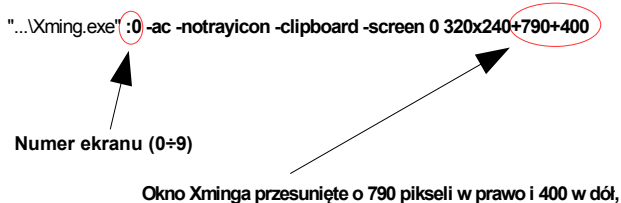
Rys. 7.41 Opis parametrów dla programu Xming.
