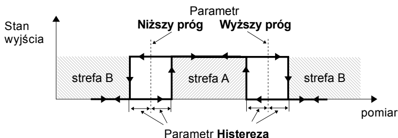
Rys. 7.89. Sterowanie dwuprogowe wyjścia przełącznikowego
