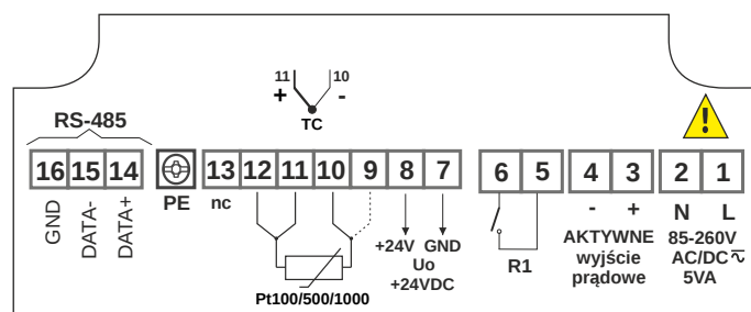
wersja z 1 x REL oraz 1 x AO 0/4-20 mA, aktywne
