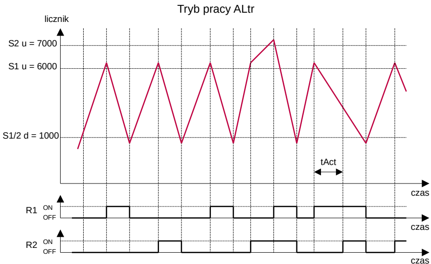
Rys. 6.10. Przebiegi obrazujące pracę przykładowego systemu
