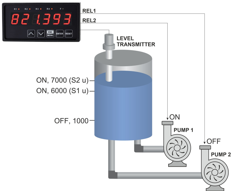
Rys. 6.9. Przykładowa konfiguracja urządzenia do sterowania pomp
