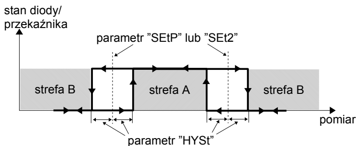
Rys. 6.4. Sterowanie dwuprogowe wyjścia przełącznikowego / diody LED
