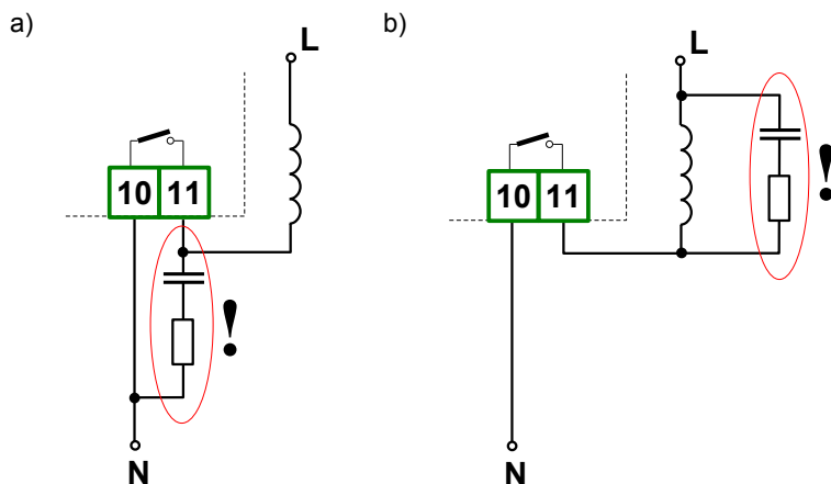
Rys. 4.10. Przykłady równoległego podłączenia obwodu tłumiącego: a) do styków przełącznika; b) do obciążenia indukcyjnego
