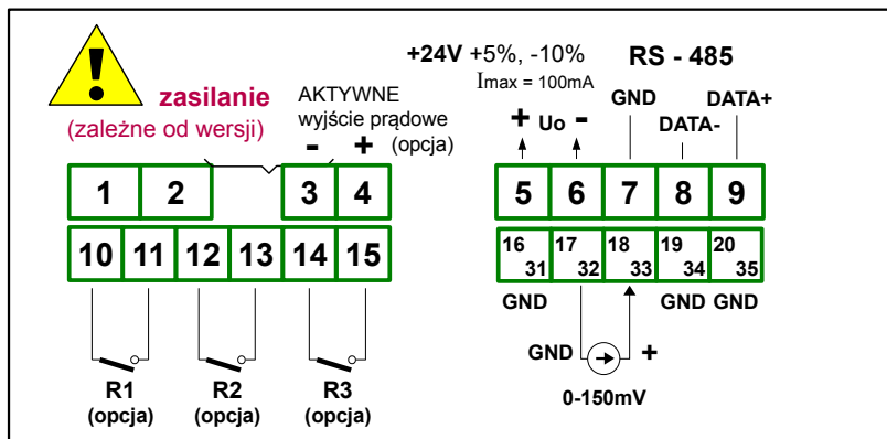
Rys. 4.7. Opis wyprowadzeń dla wersji z wyjściami przełącznikowymi oraz aktywnym wyjściem prądowym
