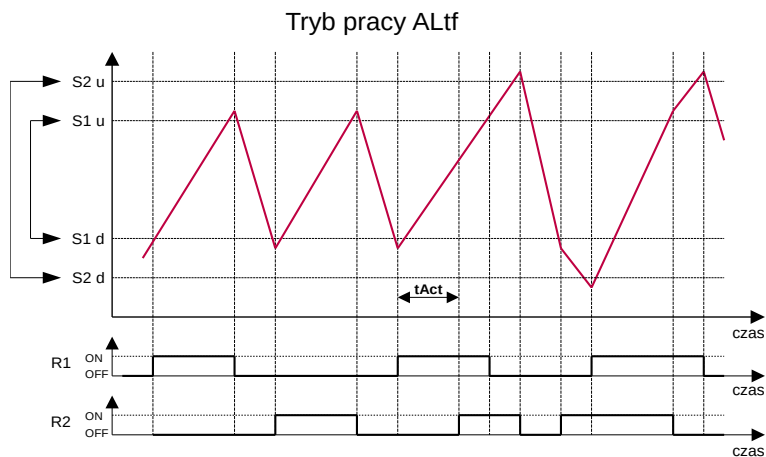
Rys. 6.6. Praca przekaźników w trybie ALtf – kontrola spadku wartości
