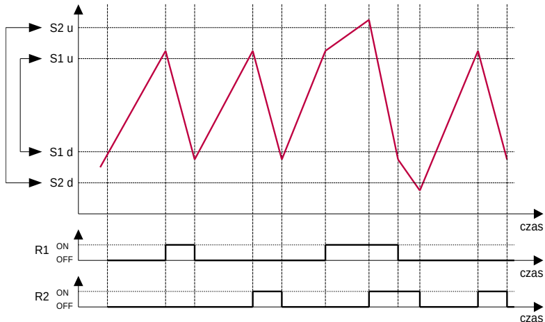
Rys. 6.5. Praca przekaźników w trybie ALtr – kontrola przyrastania wartości
