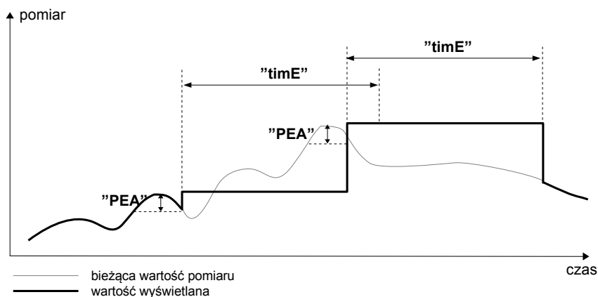
Rys. 6.3. Sposób detekcji wartości szczytowych
