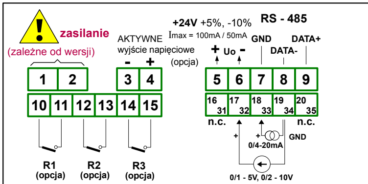
Rys. 4.12. Opis wyprowadzeń dla wersji z wyjściami przełącznikowymi oraz aktywnym wyjściem napięciowym
