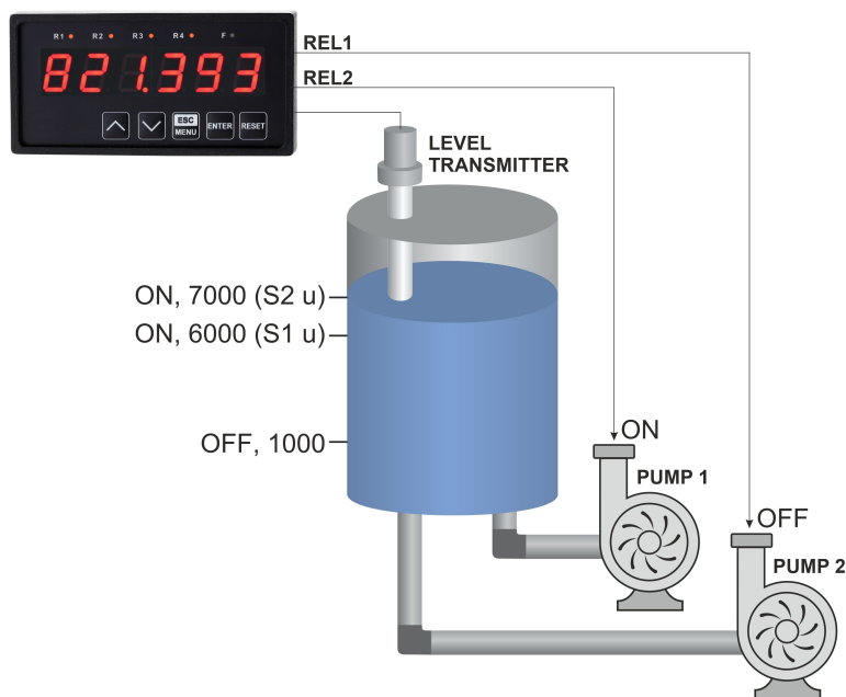
Rys. 6.11. Przykładowa konfiguracja urządzenia do sterowania pomp
