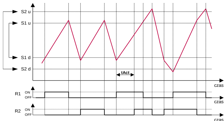
Rys. 6.8. Praca przekaźników w trybie ALTf – kontrola spadku wartości
