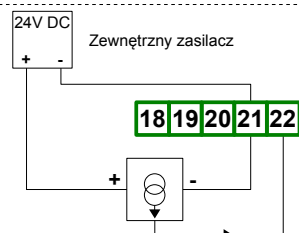
Rys. 4.12. Podłączenia przetworników prądowych 3 przewodowych
