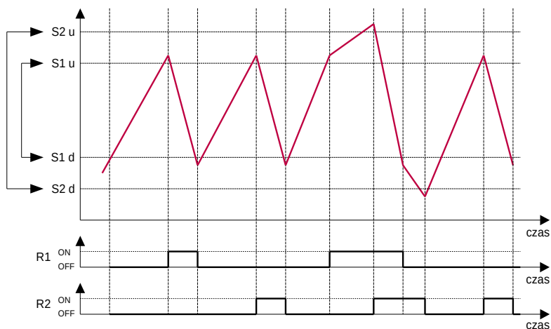
Rys. 6.7. Praca przekaźników w trybie ALTr – kontrola przystawiania wartości
