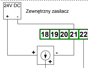
Rys. 4.13. Podłączenia przetworników napięciowych
