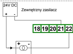
Rys. 4.11. Podłączenia przetworników prądowych 2 przewodowych
