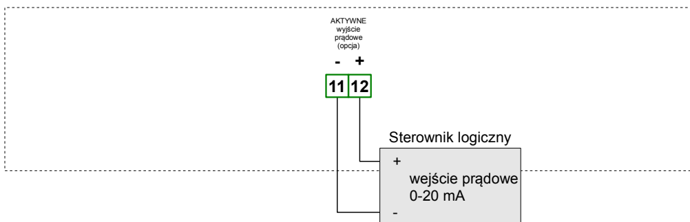
Rys. 4.18. Przykład podłączenia aktywnego wyjścia prądowego (tylko dla urządzeń posiadających aktywne wyjście prądowe)
