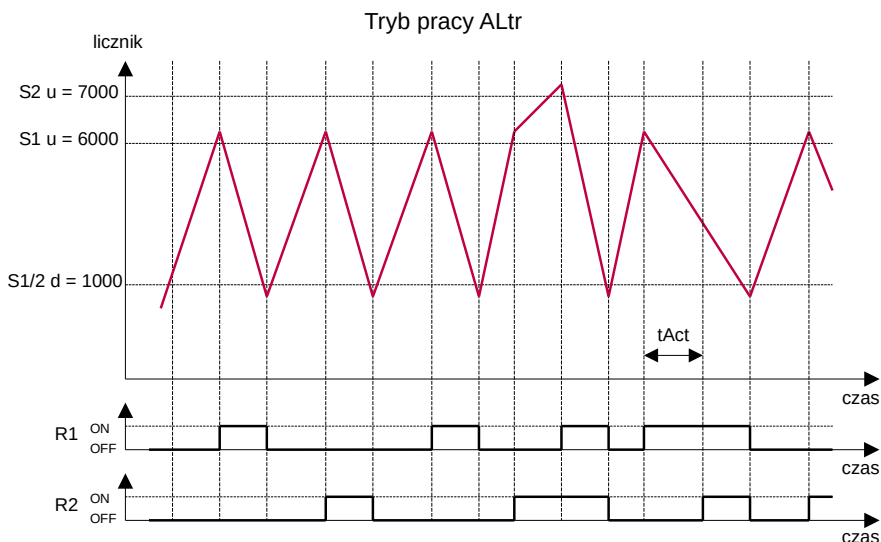
Rys. 6.12. Przebiegi obrazujące pracę przykładowego systemu
