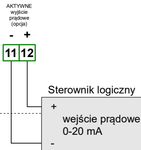
Rys. 4.17. Przykład podłączenia aktywnego wyjścia prądowego (tylko dla urządzeń posiadających aktywne wyjście prądowe)
