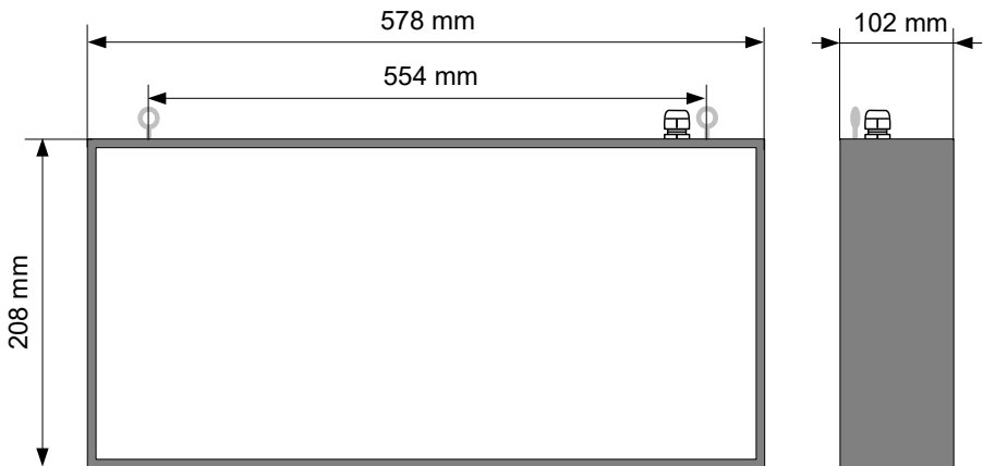
Rys. 4.1. Wymiary montażowe
