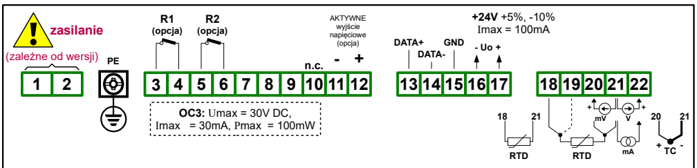
Rys. 4.9. Opis wyprowadzeń dla wersji z dwoma wyjściami przekąźnikowymi, wyjściem typu OC oraz aktywnym wyjściem napięciowym
