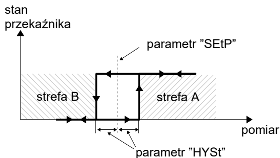
Rys. 6.5. Sterowanie jednoprogowe wyjścia przekaźnikowego
