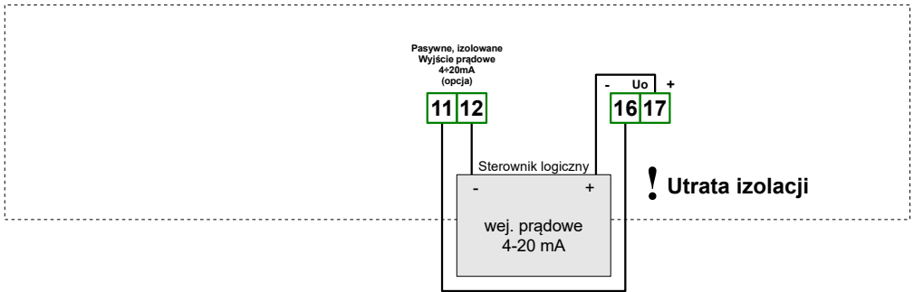
Rys. 4.18. Przykład podłączenia pasywnego wyjścia prądowego (tylko dla urządzeń posiadających pasywne wyjście prądowe)
