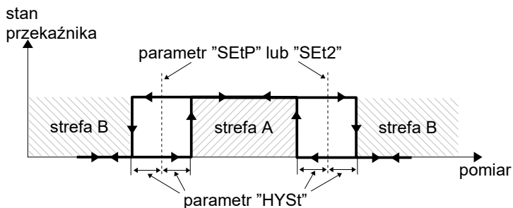
Rys. 6.6. Sterowanie dwuprogowe wyjścia przekaźnikowego
