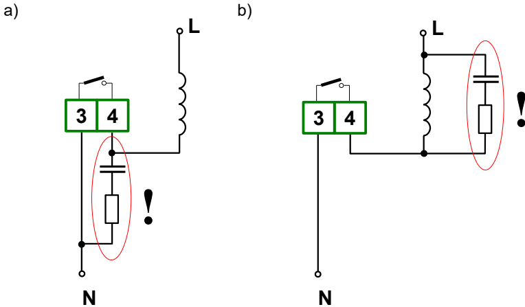
Rys. 4.15. Przykłady równoległego podłączenia obwodu tłumiącego:
