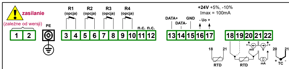
Rys. 4.5. Opis wyprowadzeń dla wersji z czterema wyjściami przełącznikowymi
