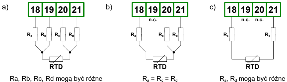
Rys. 4.13. Podłączenia zewnętrzne czujników RTD: a) 4-przewodowe; b) 3-przewodowe; c) 2-przewodowe
