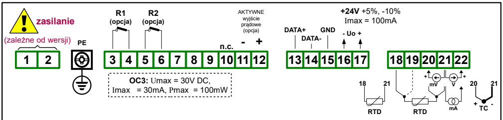
Rys. 4.8. Opis wyprowadzeń dla wersji z dwoma wyjściami przekąźnikowymi, wyjściem typu OC oraz aktywnym wyjściem prądowym
