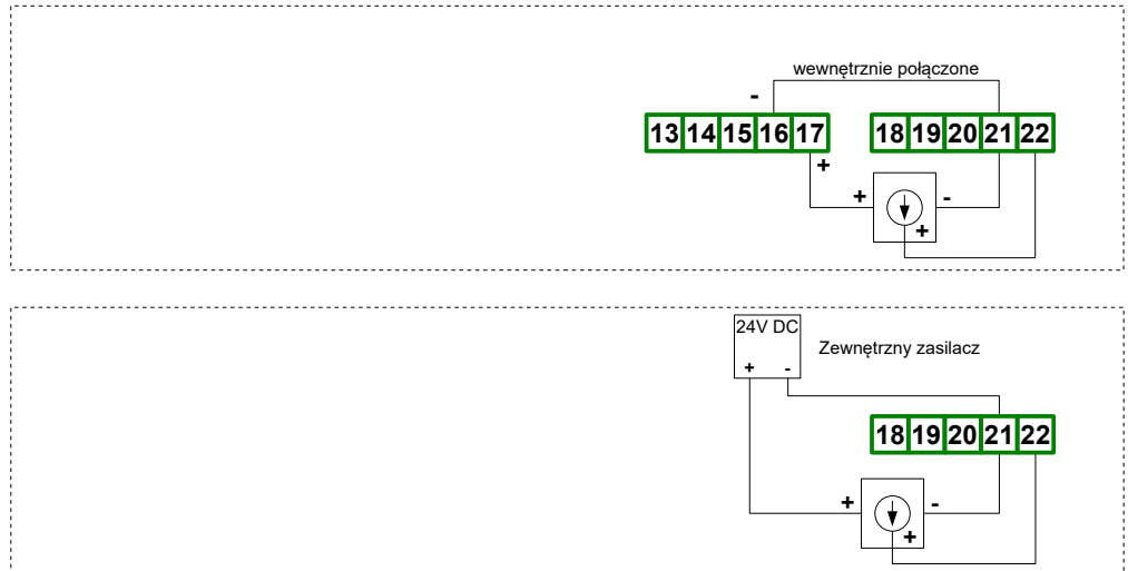
Rys. 4.12. Podłączenia przetworników napięciowych
