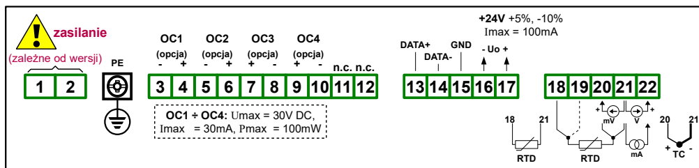
Rys. 4.6. Opis wyprowadzeń dla wersji z czterema wyjściami typu OC
