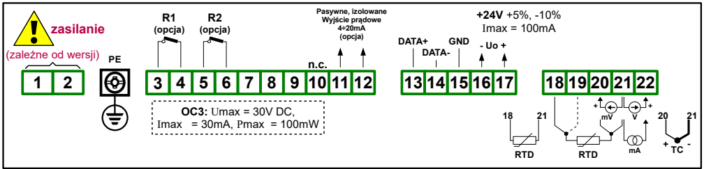
Rys. 4.7. Opis wyprowadzeń dla wersji z dwoma wyjściami przekąźnikowymi, wyjściem typu OC oraz pasywnym wyjściem prądowym
