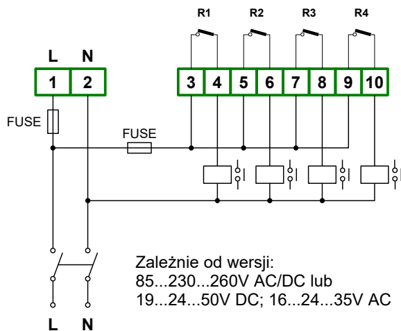
Rys. 4.14. Podłączenie zasilania oraz przekaźników sterujących obciążeniami
