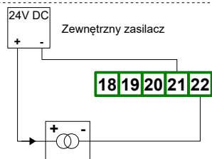
Rys. 4.10. Podłączenia przetworników prądowych 2 przewodowych
