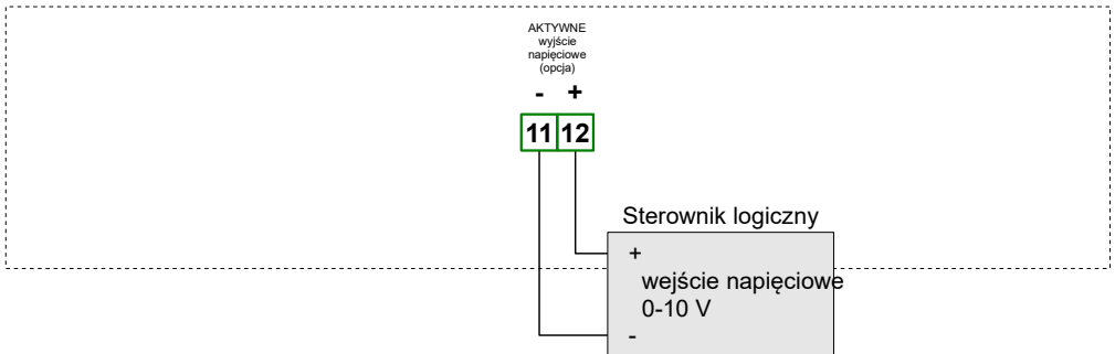
Rys. 4.19. Przykład podłączenia aktywnego wyjścia napięciowego (tylko dla urządzeń posiadających aktywne wyjście napięciowe)
