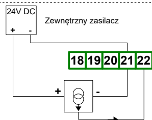
Rys. 4.11. Podłączenia przetworników prądowych 3 przewodowych
