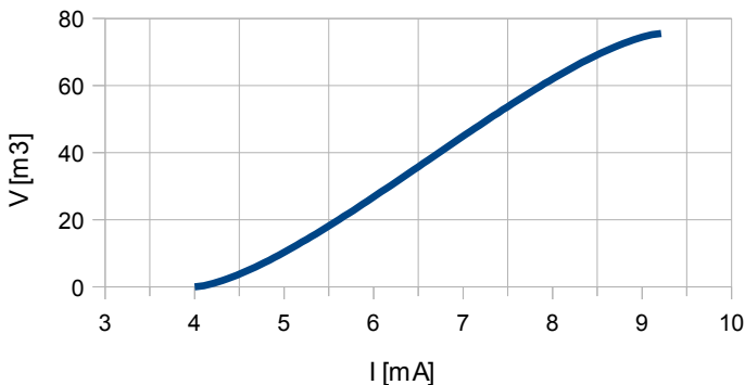
Rys. 10.7 Charakterystyka objętości zbiornika w zależności od prądu wejściowego z sondy poziomego cieczi w zbiorniku (dla zakresu 4÷20mA).
