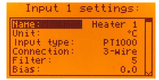
Menu "Konfiguracja wejść"
