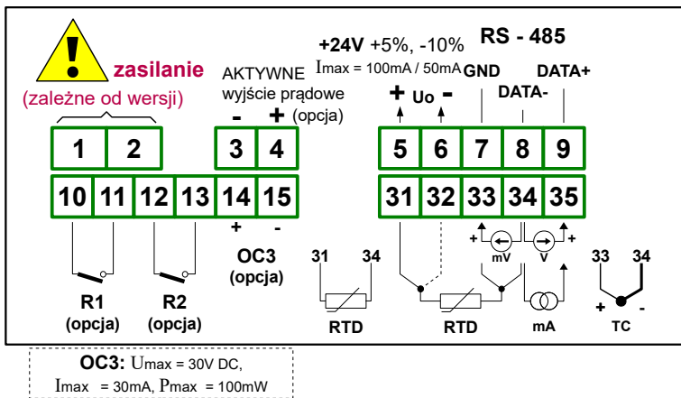
Rys. 4.9. Opis wyprowadzeń dla wersji z dwoma wyjściami przełącznikowymi, jednym wyjściem typu OC oraz aktywnym wyjściem prądowym
