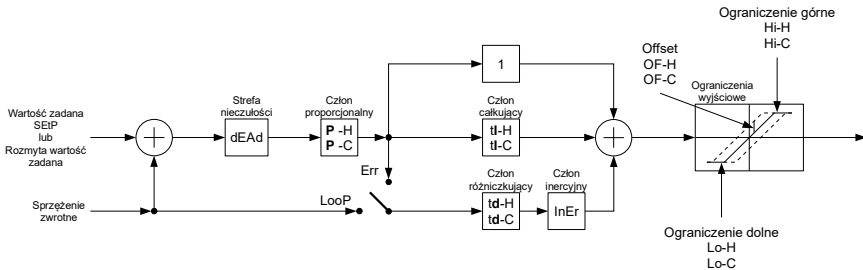
Rys. 7.2. Ogólny schemat regulatora PID zaimplementowanego w urządzeniu PUR-49D
