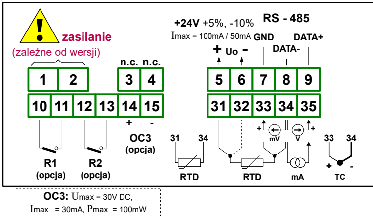
Rys. 4.8. Opis wyprowadzeń dla wersji z dwoma wyjściami przełącznikowymi oraz wyjściem typu OC
