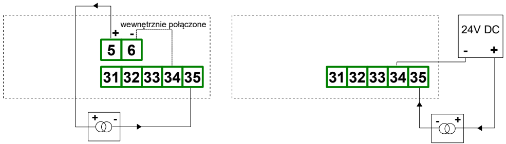
Rys. 4.12. Podłączenia przetworników prądowych 2 przewodowych
