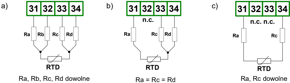
Rys. 4.15. Podłączenia zewnętrzne czujników RTD: a) 4-przewodowe; b) 3-przewodowe; c) 2-przewodowe
