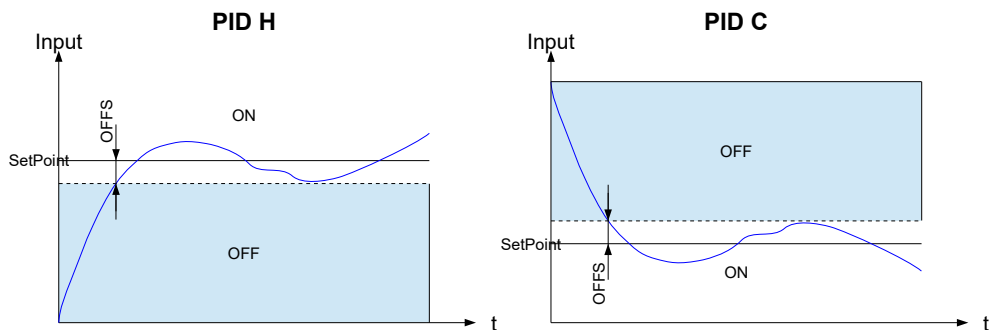
Rys. 6.7. Charakterystyki sterowania przełącznika w zależności od trybu pracy
