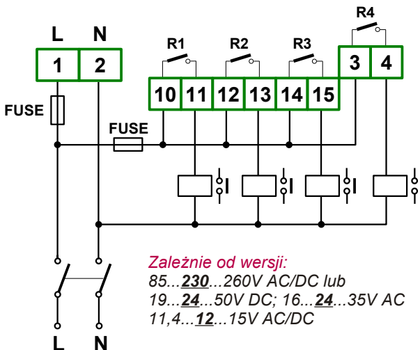
Rys. 4.16. Podłączenie zasilania oraz przekaźników sterujących obciążeniami
