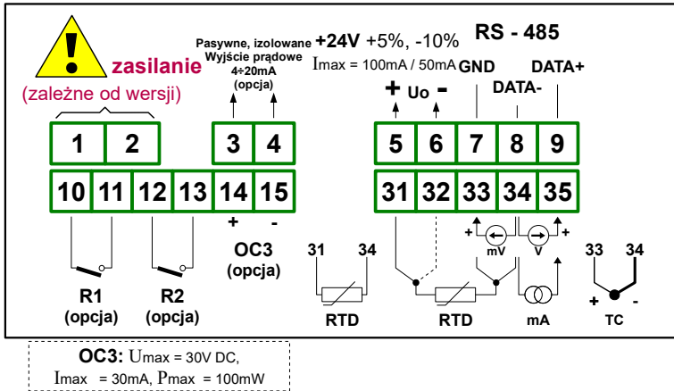
Rys. 4.10. Opis wyprowadzeń dla wersji z dwoma wyjściami przełącznikowymi, jednym wyjściem typu OC oraz pasywnym wyjściem prądowym
