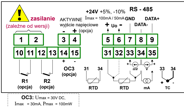
Rys. 4.11. Opis wyprowadzeń dla wersji z dwoma wyjściami przełącznikowymi, jednym wyjściem typu OC oraz aktywnym wyjściem napięciowym
