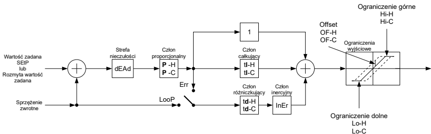
Rys. 6.6. Ogólny schemat regulatora PID zaimplementowanego w urządzeniu PUR-49D
