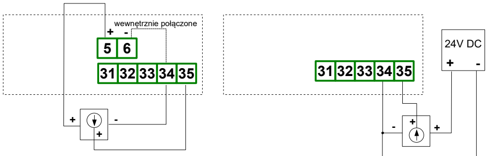
Rys. 4.14. Podłączenia przetworników napięciowych
