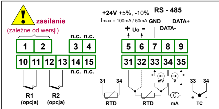
Rys. 4.5. Opis wyprowadzeń dla wersji z dwoma wyjściami przełącznikowymi
