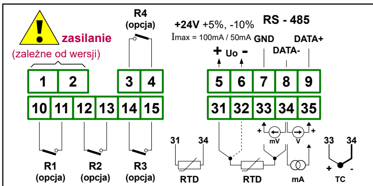
Rys. 4.7. Opis wyprowadzeń dla wersji z czterema wyjściami przełącznikowymi
