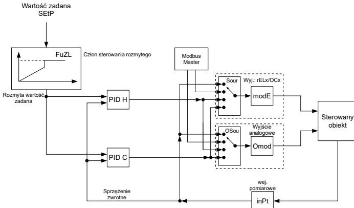
Rys. 6.5 Struktura ogólna urządzenia PUR-49D
