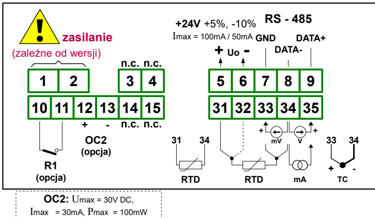
Rys. 4.6. Opis wyprowadzeń dla wersji z wyjściem przełącznikowym i wyjściem typu OC
