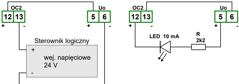
Rys. 4.18. Przykładowe podłączenia wyjścia typu OC (tylko dla urządzeń posiadających wyjście typu OC)
