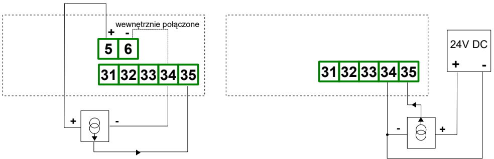
Rys. 4.13. Podłączenia przetworników prądowych 3 przewodowych
