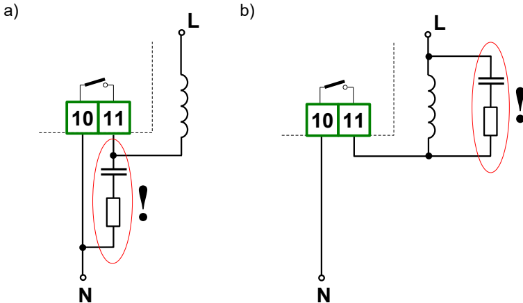
Rys. 4.17. Przykłady równoległego podłączenia obwodu tłumiącego: a) do styków przekaźnika; b) do obciążenia indukcyjnego
