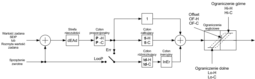
Rys. 6.6. Ogólny schemat regulatora PID zaimplementowanego w urządzeniu PUR-94D
