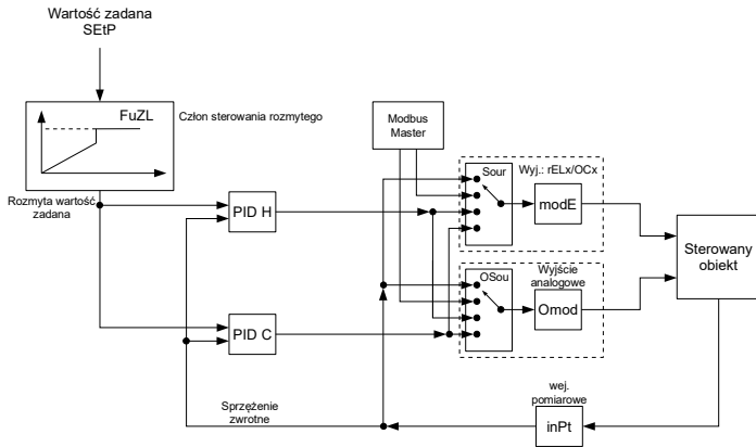
Rys. 6.5 Struktura ogólna urządzenia PUR-94D
