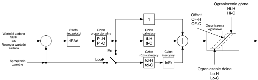
Rys. 7.2. Ogólny schemat regulatora PID zaimplementowanego w urządzeniu PUR-94D
