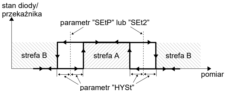
Rys. 6.11. Sterowanie dwuprogowe wyjścia przełącznikowego / diody LED
