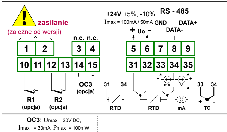
Rys. 4.9. Opis wyprowadzeń dla wersji z dwoma wyjściami przekąźnikowymi oraz wyjściem typu OC
