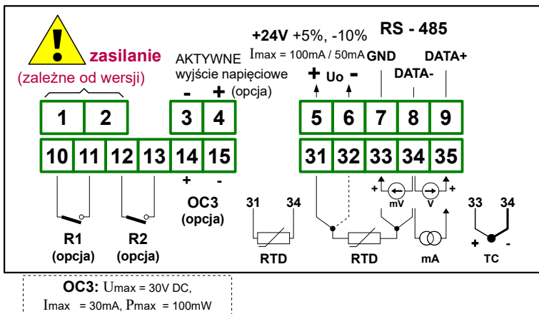
Rys. 4.12. Opis wyprowadzeń dla wersji z dwoma wyjściami przełącznikowymi, jednym wyjściem typu OC oraz aktywnym wyjściem napięciowym
