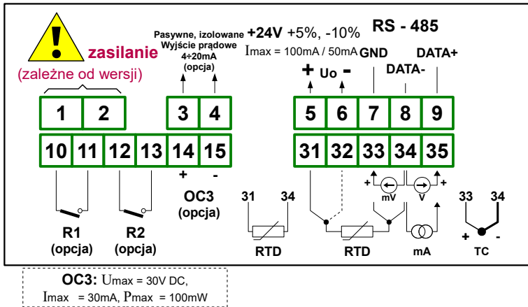
Rys. 4.11. Opis wyprowadzeń dla wersji z dwoma wyjściami przełącznikowymi, jednym wyjściem typu OC oraz pasywnym wyjściem prądowym
