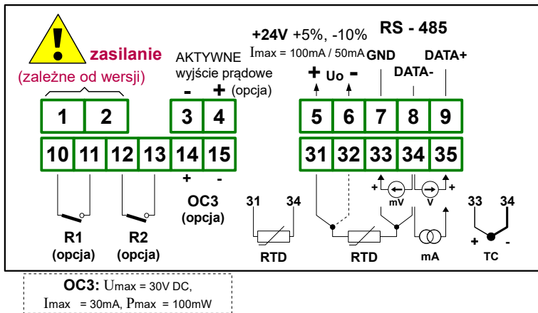
Rys. 4.10. Opis wyprowadzeń dla wersji z dwoma wyjściami przekąźnikowymi, jednym wyjściem typu OC oraz aktywnym wyjściem prądowym
