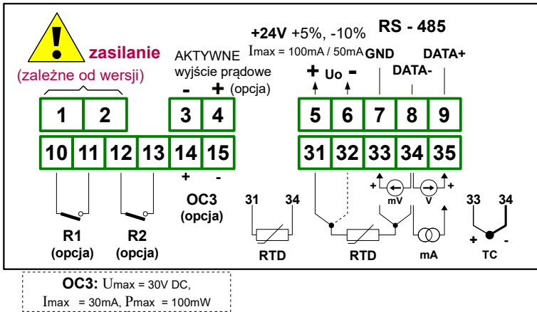
Rys. 4.9. Opis wyprowadzeń dla wersji z dwoma wyjściami przekaźnikowymi, jednym wyjściem typu OC oraz aktywnym wyjściem prądowym
