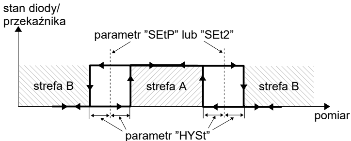
Rys. 6.6. Sterowanie dwuprogowe wyjścia przełącznikowego / diody LED
