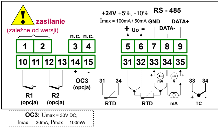
Rys. 4.8. Opis wyprowadzeń dla wersji z dwoma wyjściami przekaźnikowymi oraz wyjściem typu OC
