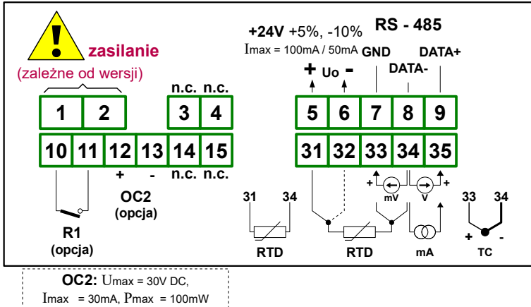
Rys. 4.6. Opis wyprowadzeń dla wersji z wyjściem przekaźnikowym i wyjściem typu OC
