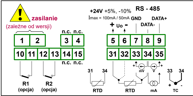
Rys. 4.5. Opis wyprowadzeń dla wersji z dwoma wyjściami przekaźnikowymi
