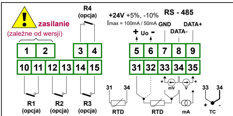
Rys. 4.7. Opis wyprowadzeń dla wersji z czterema wyjściami przekaźnikowymi
