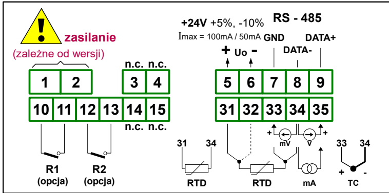
Rys. 4.6. Opis wyprowadzeń dla wersji z dwoma wyjściami przekaźnikowymi
