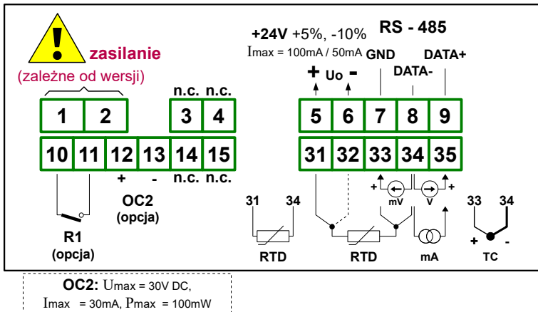
Rys. 4.7. Opis wyprowadzeń dla wersji z wyjściem przekaźnikowym i wyjściem typu OC
