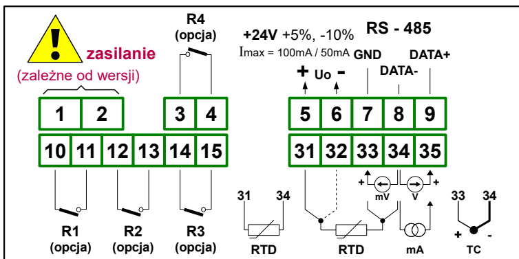
Rys. 4.8. Opis wyprowadzeń dla wersji z czterema wyjściami przekaźnikowymi
